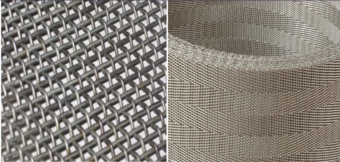
Woven FeCrAl Mesh
